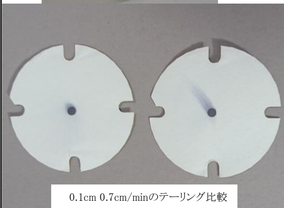
②一定時間静止し引き上げる。ペーパーに発生した尾引き(テーリング)の長さ と方位を専用定規で読み取り流向流速に変換
