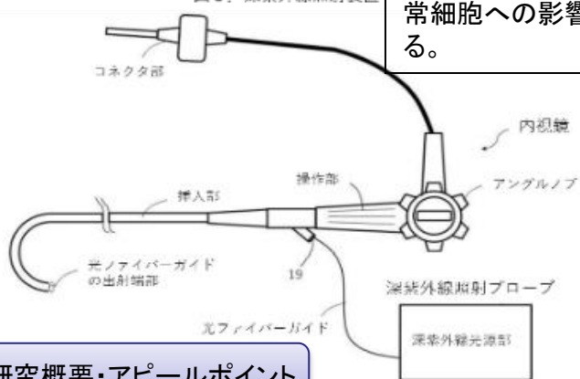
図3. 深紫外線照射装置
