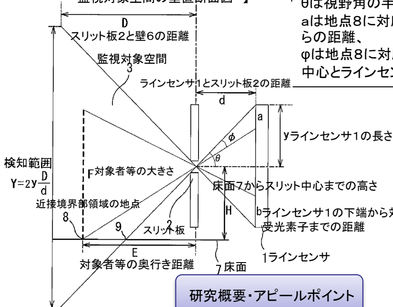
【 一次元輝度分布検知装置及び監視対象空間の垂直断面図 】
