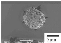
高分子多孔質粒子の走査型イオン顕微鏡写真
