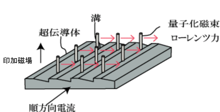
【図1】溝状人工ピンの基本的形態を示す図
