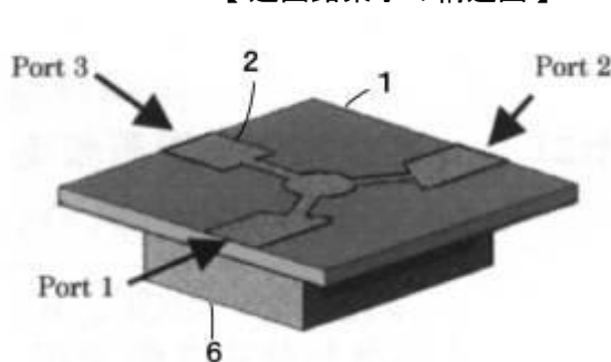
【逆回路素子の構造図】
