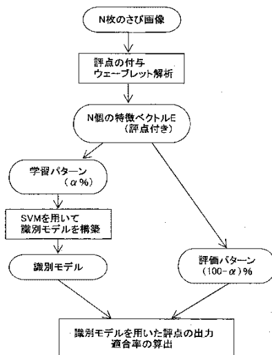
【構築される識別モデルの有効性を検証する過程図】
