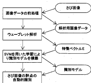
【識別の過程を示すフロー図】
