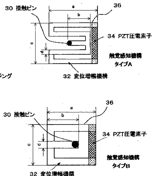
(b) 触覚感知機構を示す図
