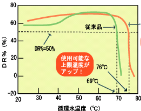
本発明の実施例における最大DRR(%)と循環水温度との関係を示すグラフ
